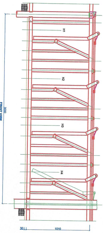
معالف أبقار موديل (HLK43) 4 رؤس كل 3 أمتار HEADLOCKS MODEL (HLK43)
